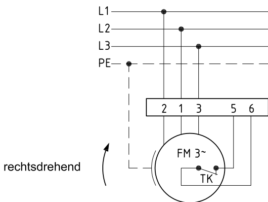
Anschlußplan 0.13-2 r.
