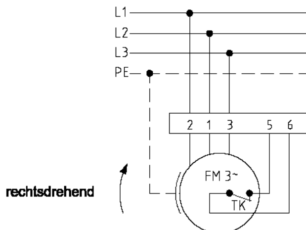
Anschlußplan 0.13-2 r.
