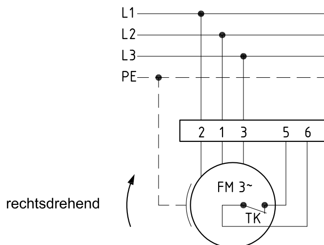
Anschlußplan 0.13-2 r.
